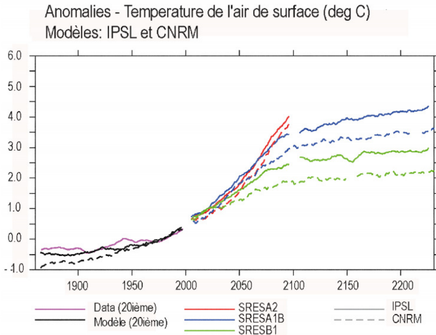
Figure 8 : Variation de la température moyenne de surface de 1850 à 2200 pour 3 scénarios (A2, A1B et B1) d'émissions de gaz à effet de serre (Copyright Météo-France / IPSL, 2007)
